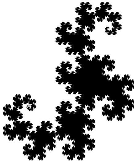
FIGURE II.8 – Dragon gauche de profondeur 15
